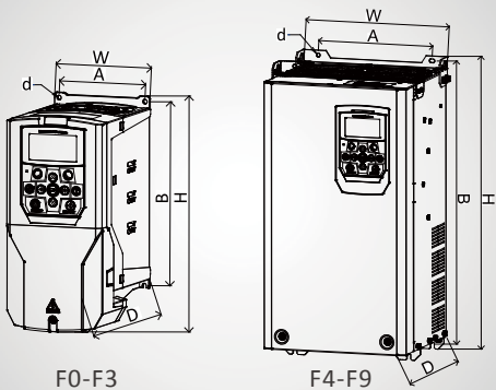
ES系列塑胶/钣金结构外形尺寸及安装示意图
