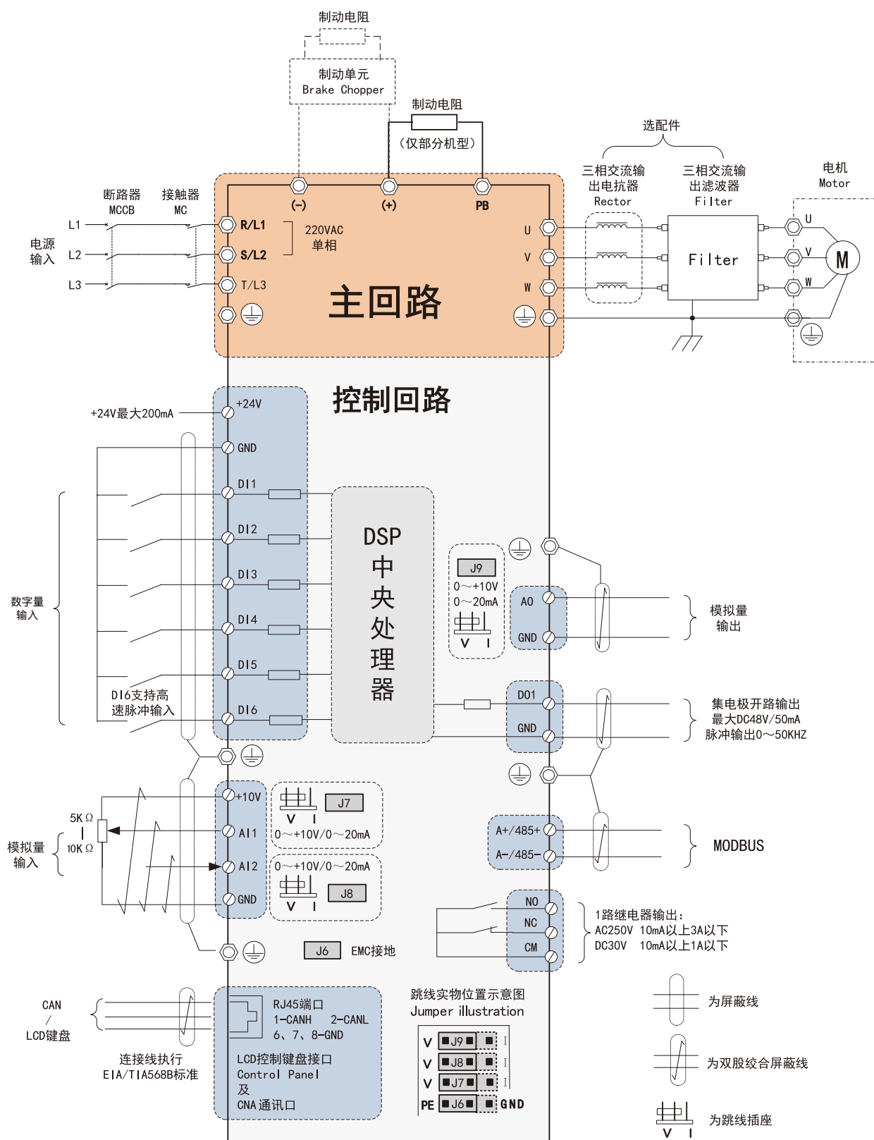
标准接线图2(适用于F0)
