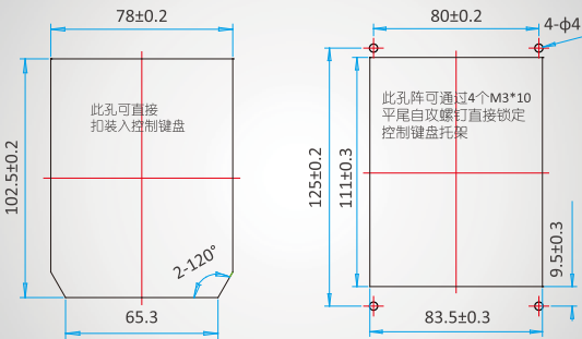
控制键盘/托架直接门上安装开孔形状与尺寸图
