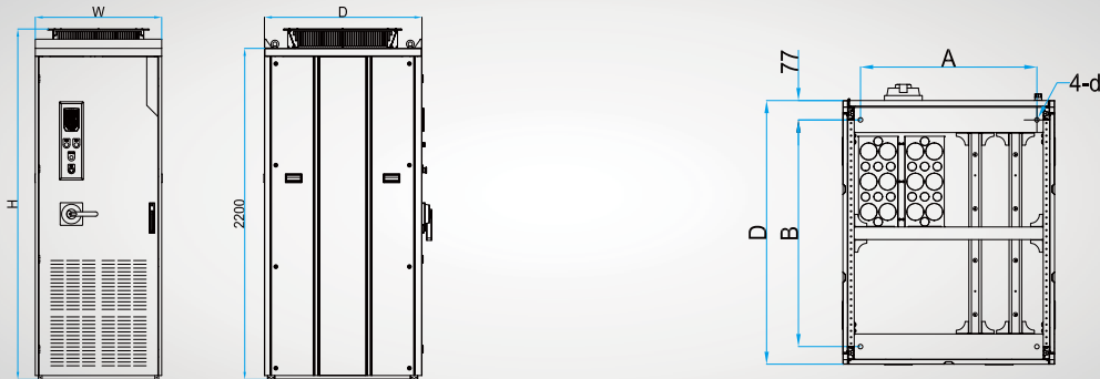
C10及以上柜体机结构外形尺寸及安装示意图
