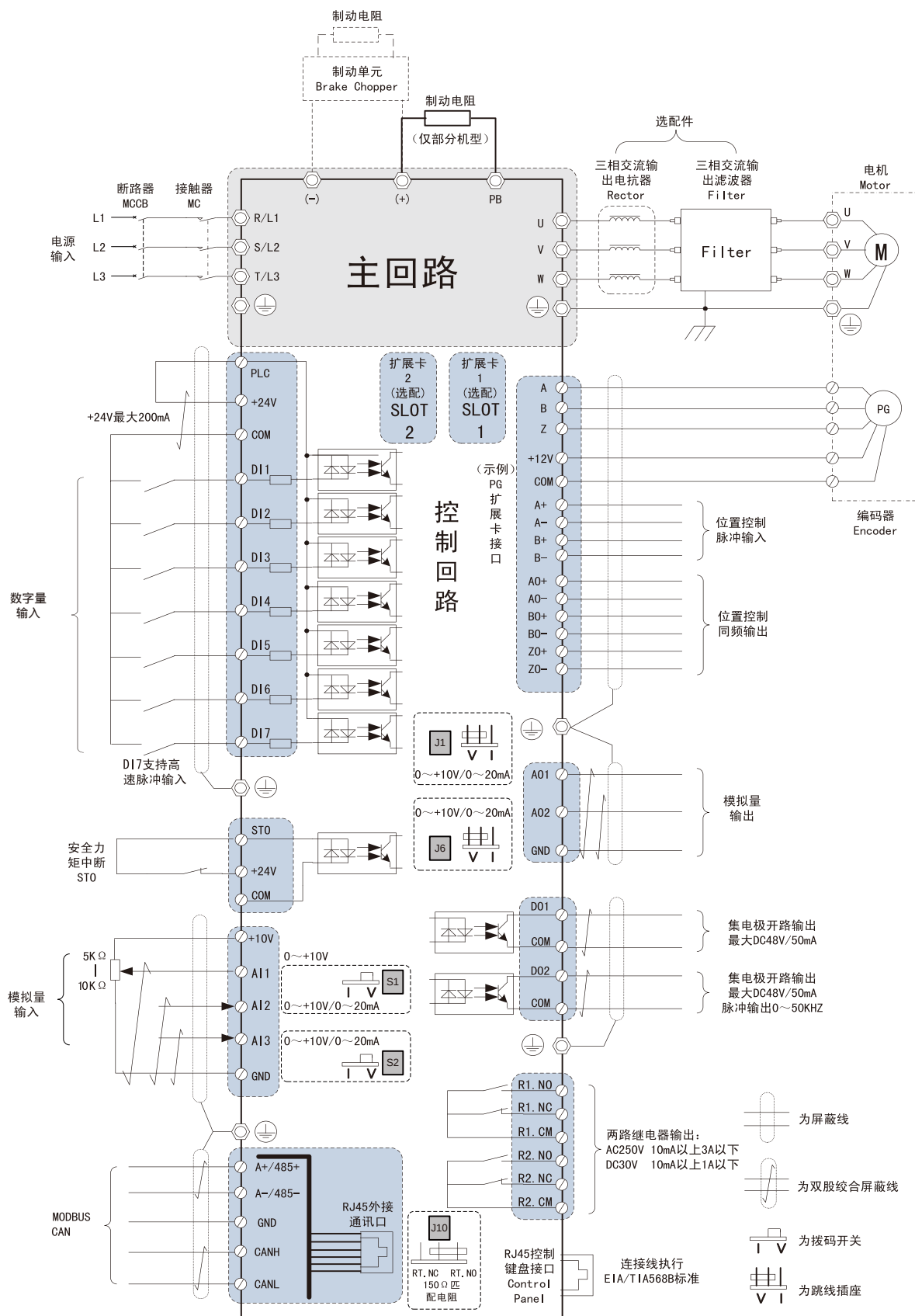
标准接线图1(适用于F1及以上)
